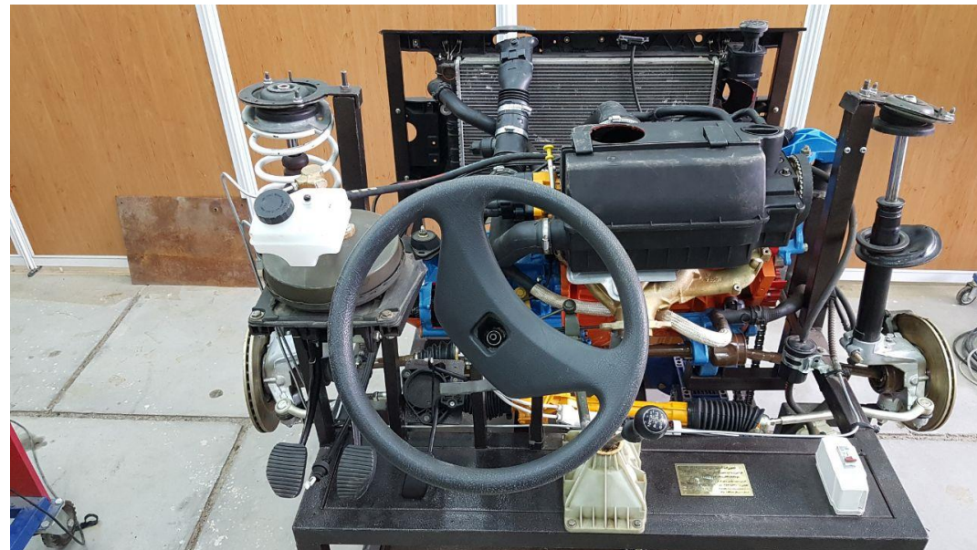
استند موتور و گیربکس پژه ۴۰۵ (برش خورده)
